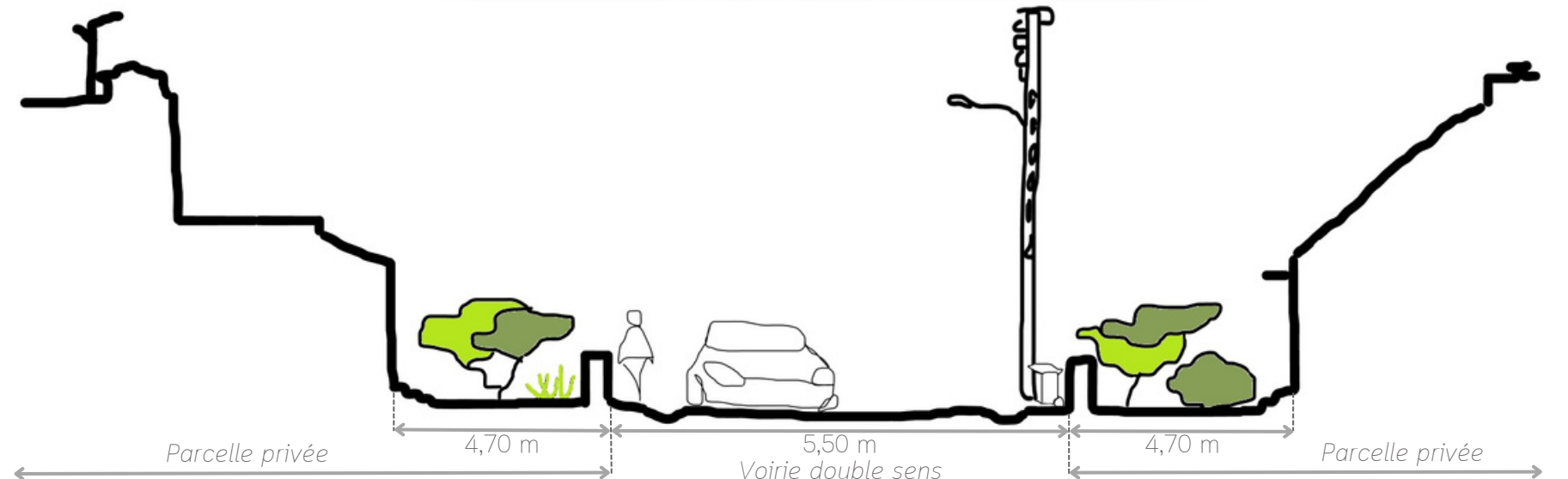
Coupe de la rue du Cambodge
